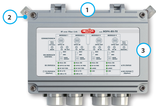
mod. ROF4-RX-TX
