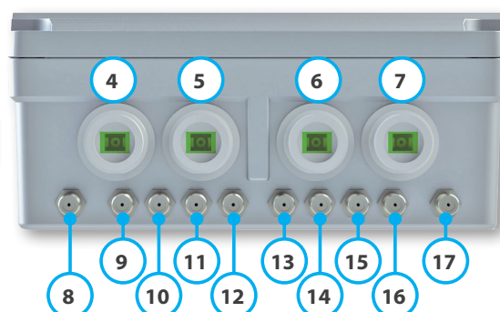
mod. ROF4-RX-TX
