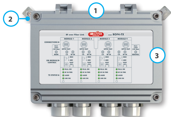
mod. ROF4-TX
