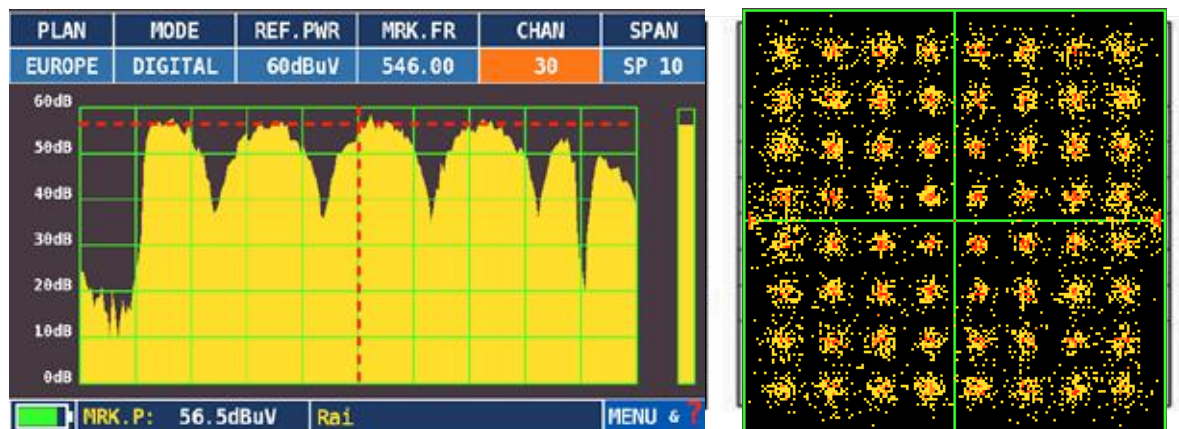
Fig.1 vediamo lo spettro di un segnale di livello buono con a fianco l'immagine della costellazione che mostra una lieve degradazione
