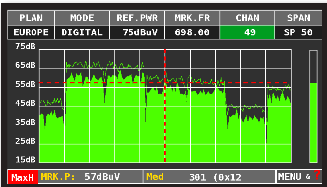
Spettro veloce con memoria di picco "MAX H"
