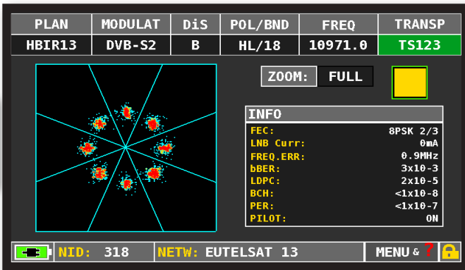
Costellazione 8PSK.
