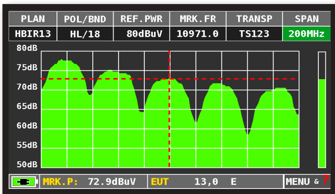
Spettro veloce
